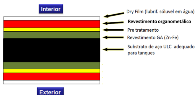
Figura 2 – Camadas na formação do aço para estampagem (Carvalho et al., 2009).
