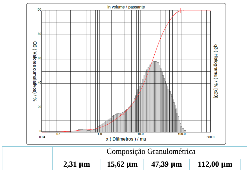
Figura 1: Determinação da distribuição de tamanhos de partículas.
