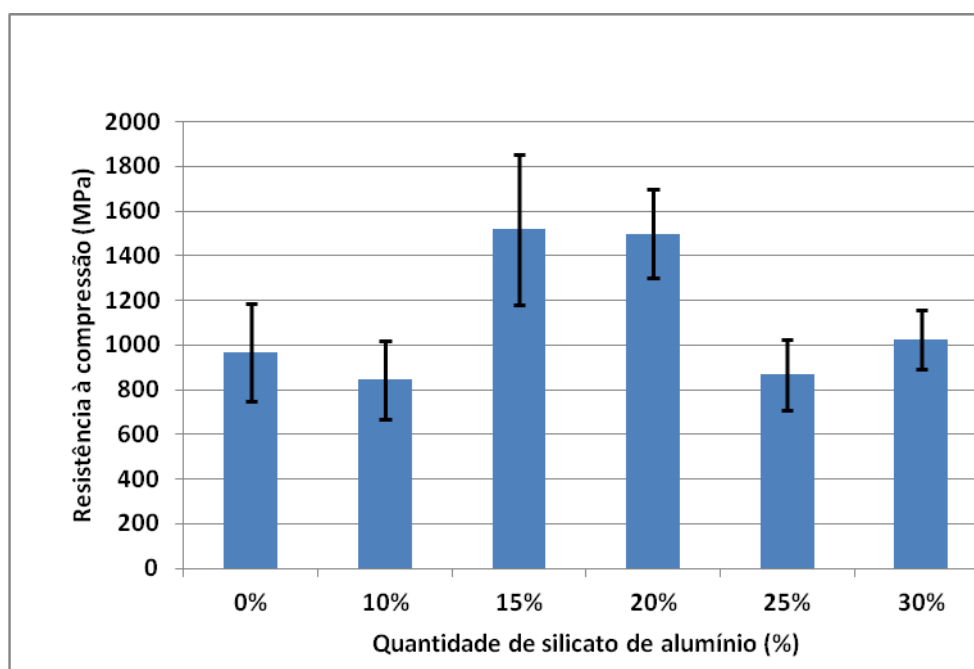
Figura 7: Ensaios de resistência à compressão dos corpos de prova.
