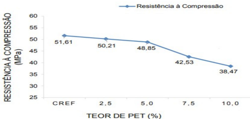
Figura 4 – Resultados: resíduos de PET
