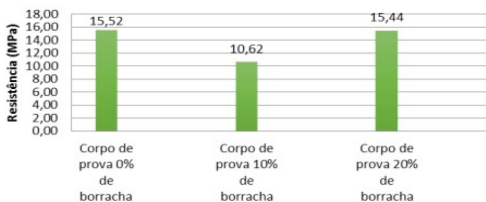
Figura 2 – Resultados: resíduos de borrachas de pneus
