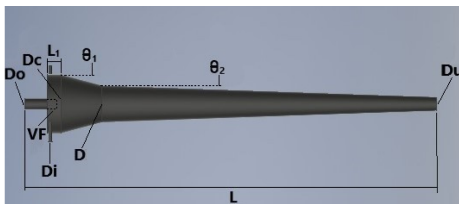
Figura 1: Protótipo de um hidrociclone para separação óleo-água.
