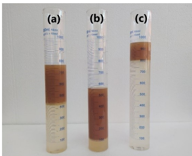
Figura 4: Amostras da mistura óleo-água recolhidas na entrada (a), overflow (b) e underflow (c) com Razão de Fluido 32% para o Experimento 1.
